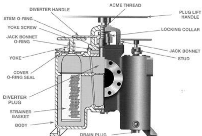
Изображение основных компонентов Дуплексная модель 50
